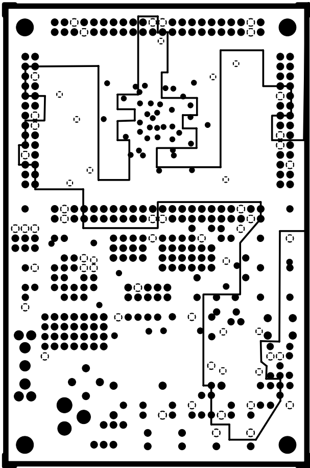
V33 VCCINT
