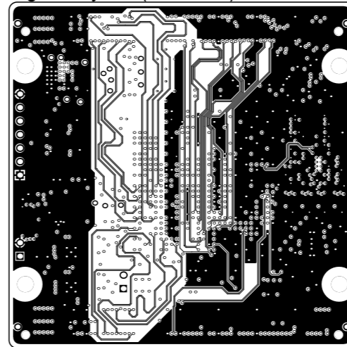
Signal Layer 5 (Scale 1:1)
