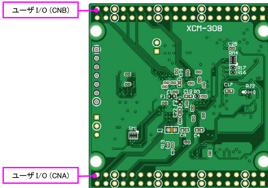
はんだ面
