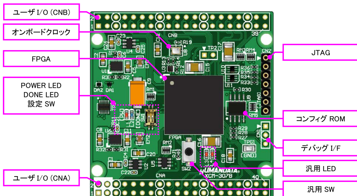
部品面
