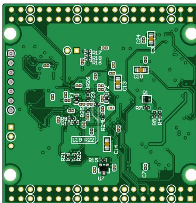
はんだ面
