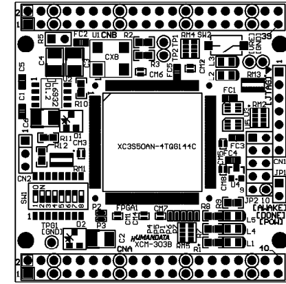
部品面
