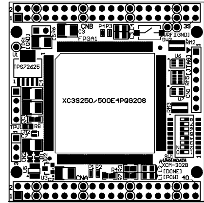
部品面
