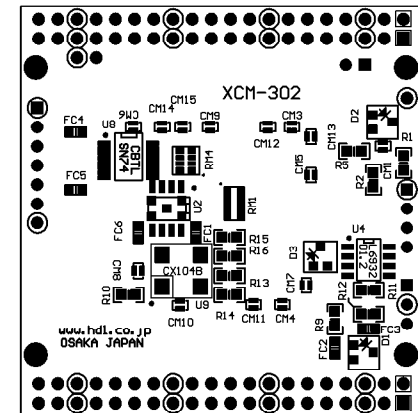
はんだ面
