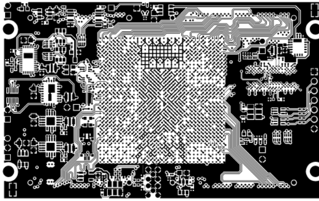
TOP LAYER
