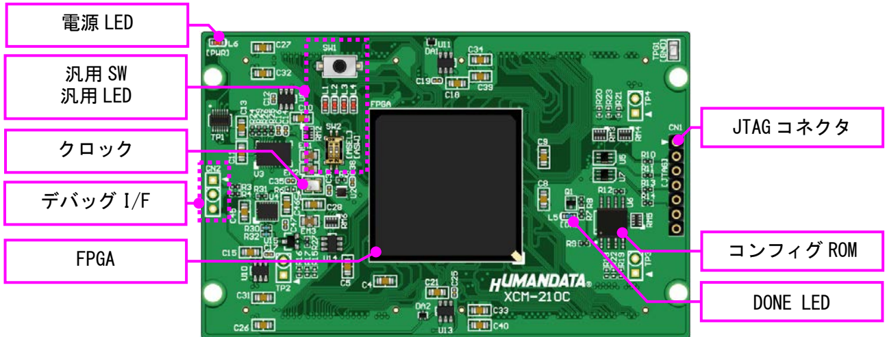
部品面
