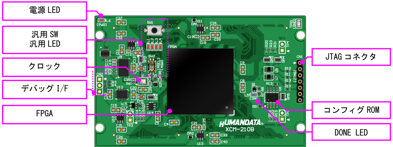
部品面
