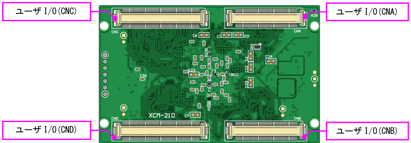
はんだ面
