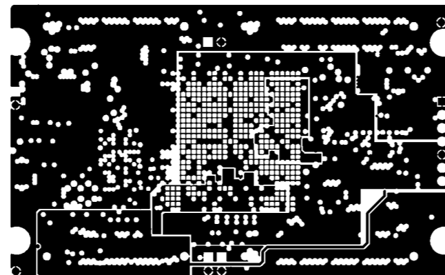
MID LAYER 6
