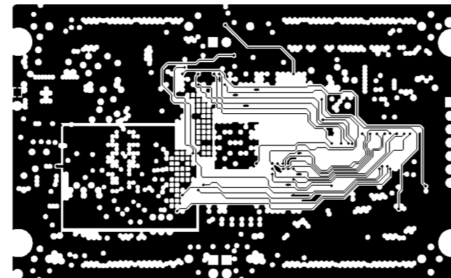
MID LAYER 5
