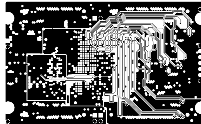
MID LAYER 4
