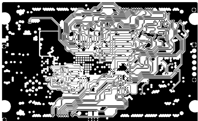
MID LAYER 2
