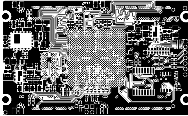
TOP LAYER
