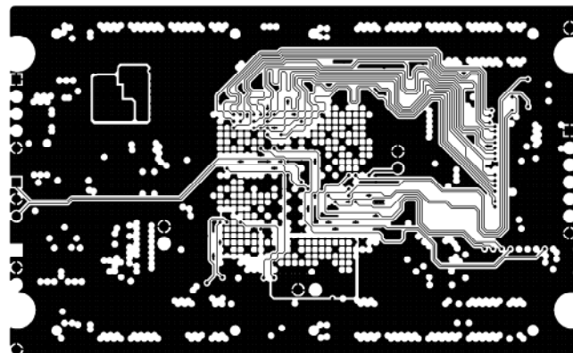
MID LAYER 3
