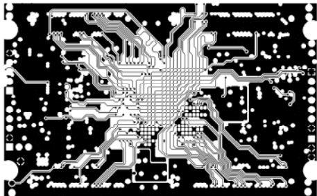
MID LAYER 1
