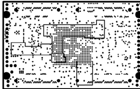
MID LAYER 4
