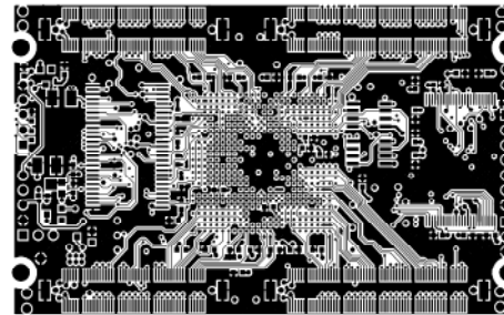
BOTTOM LAYER
