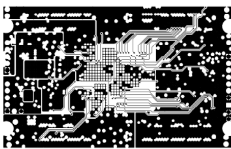
MID LAYER 4
