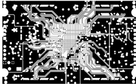
MID LAYER 2
