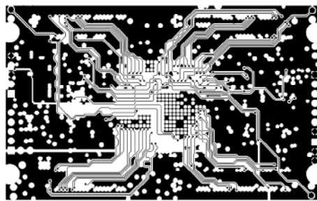
MID LAYER 3
