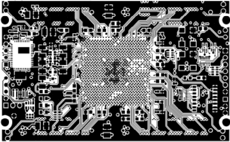
TOP LAYER
