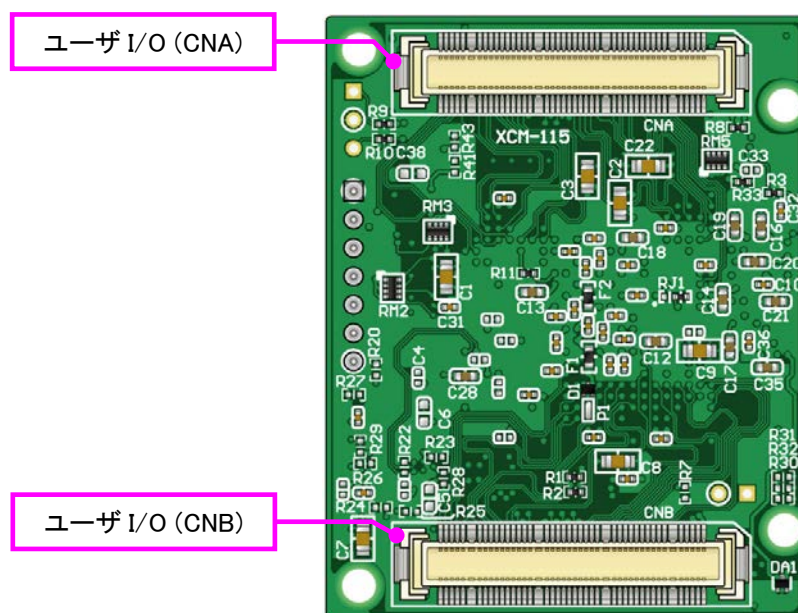
はんだ面
