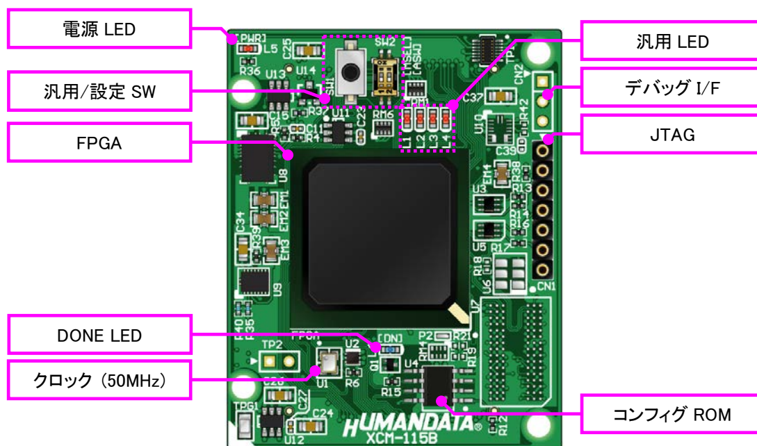
部品面
