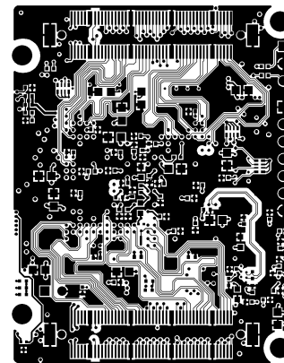
BOTTOM LAYER
