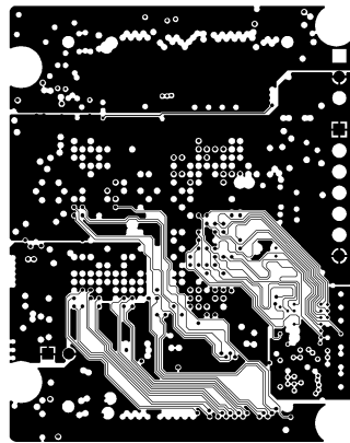
MID LAYER 2
