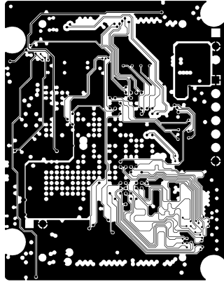
MID LAYER 1
