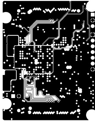
MID LAYER 3
