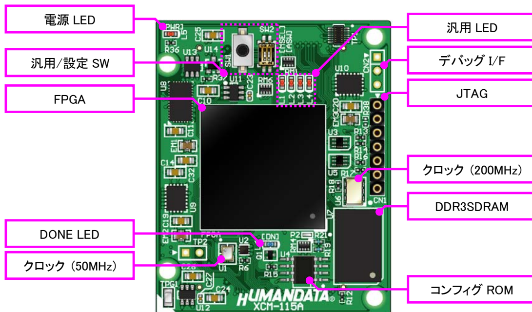
部品面
