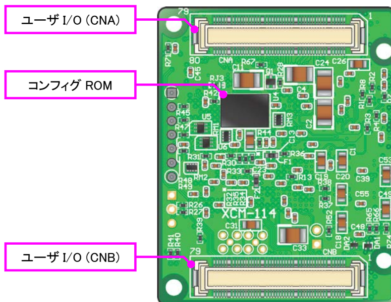
はんだ面
