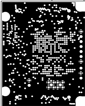
InternalPlane1 (Scale 1:1)
