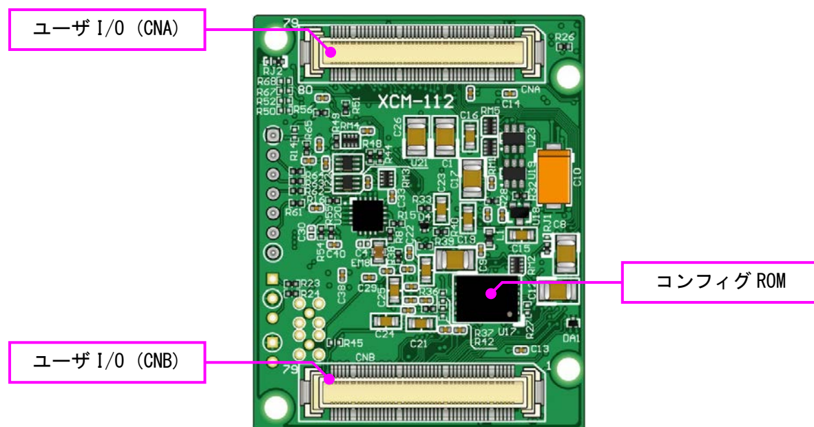
はんだ面
