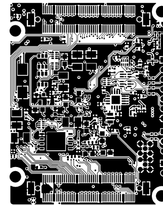
BOTTOM LAYER
