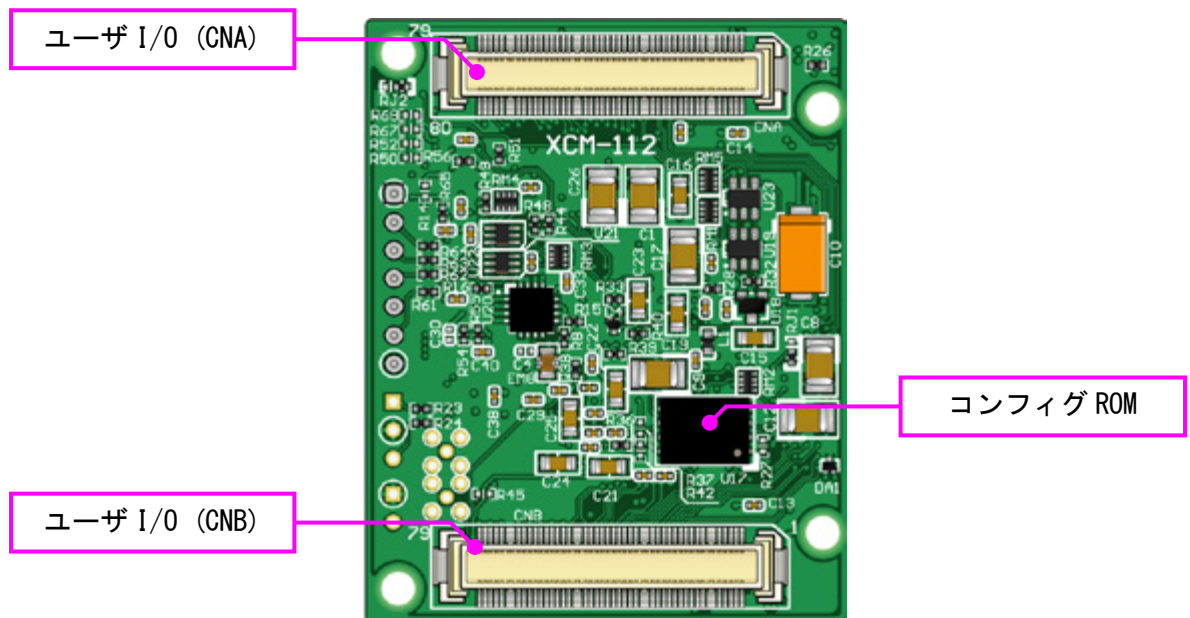
はんだ面
