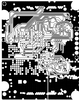
MID LAYER2
