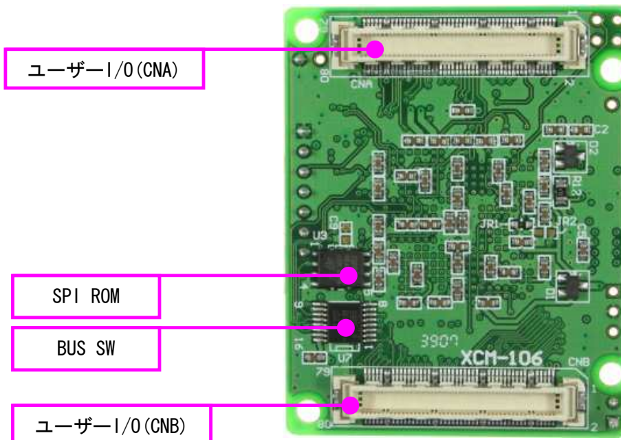
<はんだ面>
