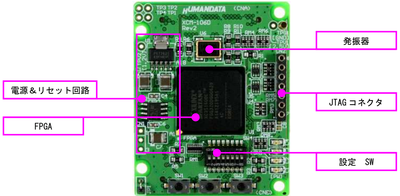
<部品面>
