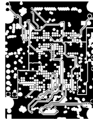
MID LAYER2
