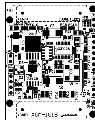
部品面
