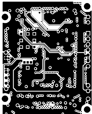
MID LAYER2
