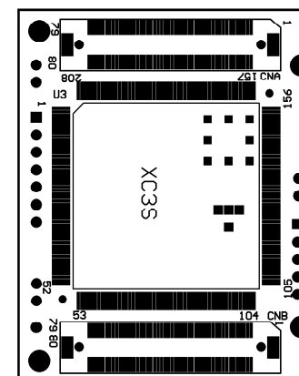
はんだ面
