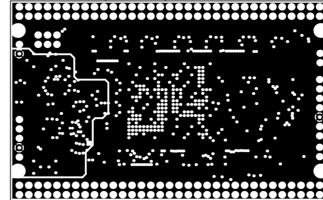
InternalPlane2 (Scale 1:1)
