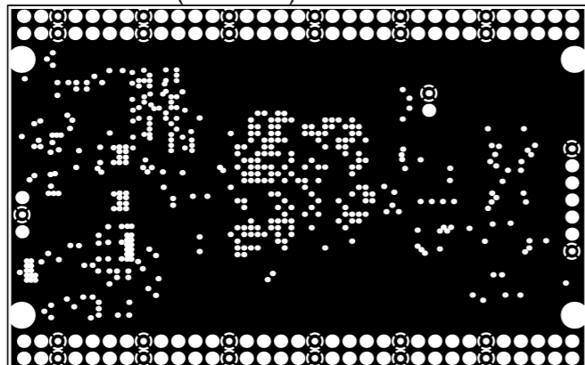
InternalPlane1 (Scale 1:1)
