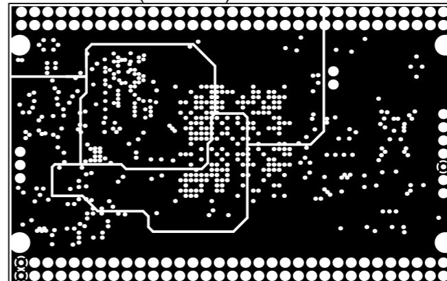
InternalPlane2 (Scale 1:1)
