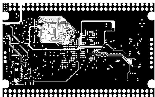
MID LAYER1
