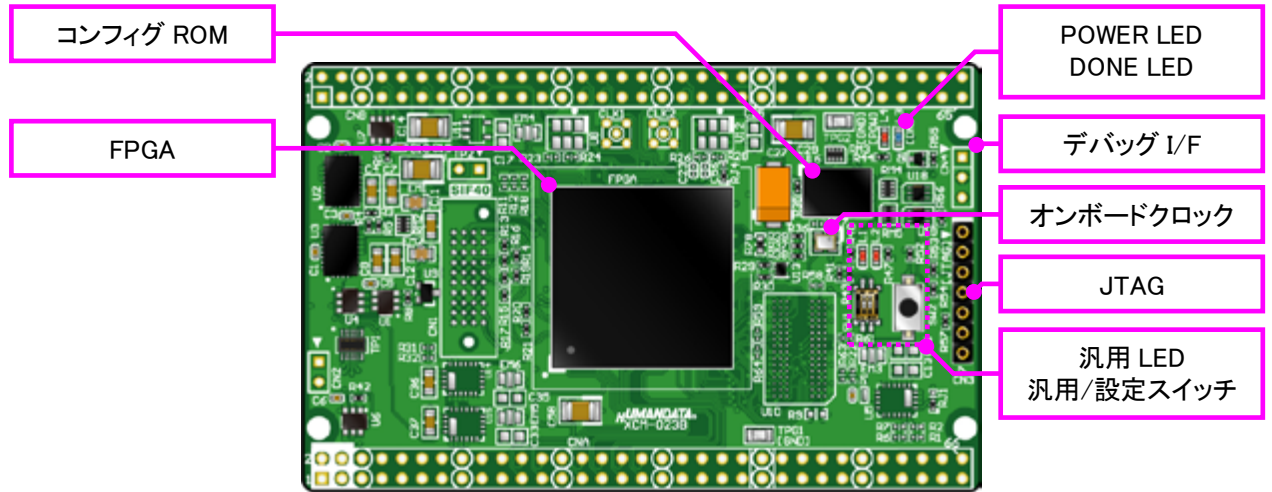
部品面
