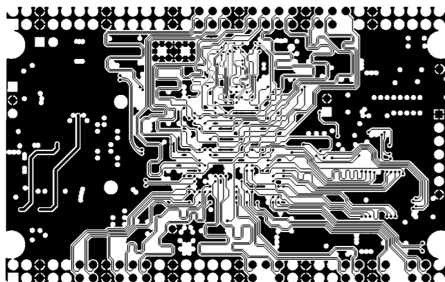
MID LAYER1
