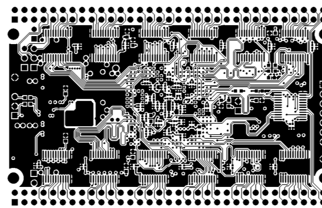
BOTTOM LAYER
