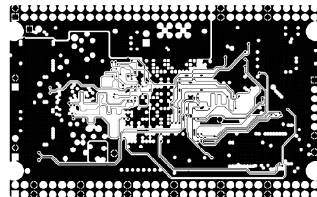
MID LAYER2
