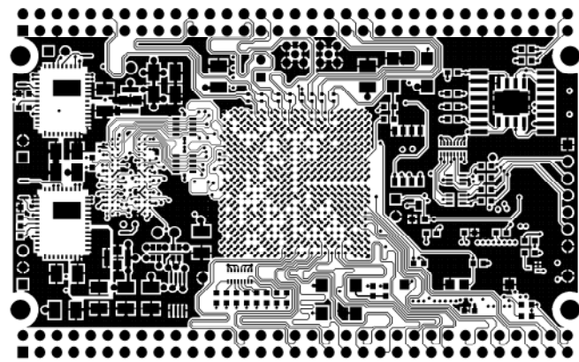
TOP LAYER
