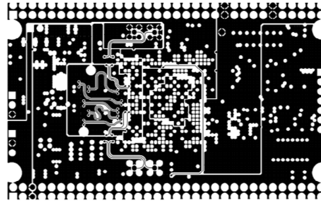
MID LAYER2
