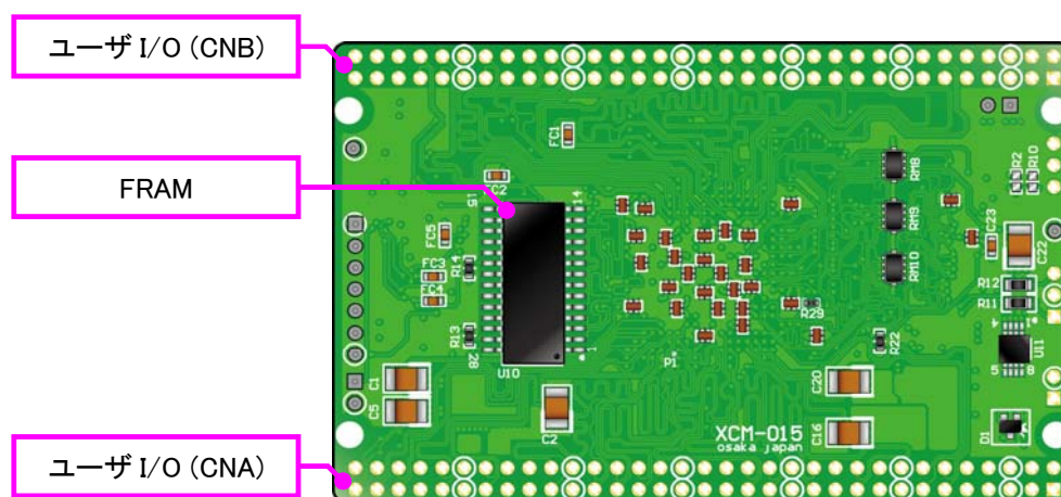
はんだ面
