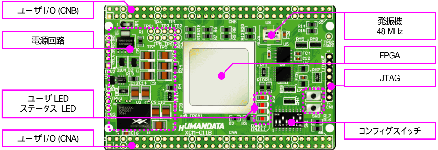
部品面
