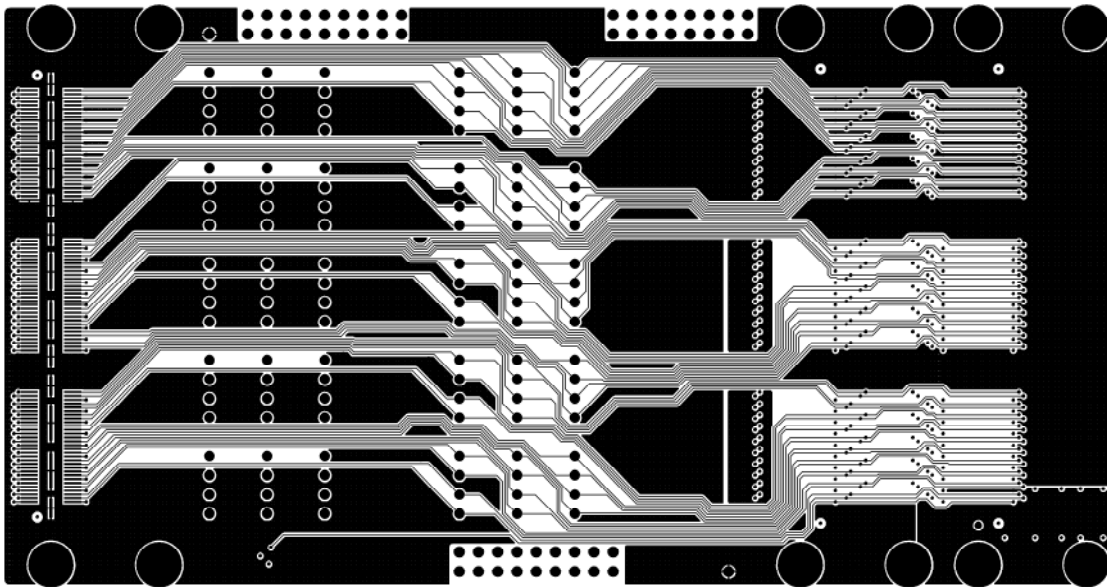
BOTTOM LAYER
