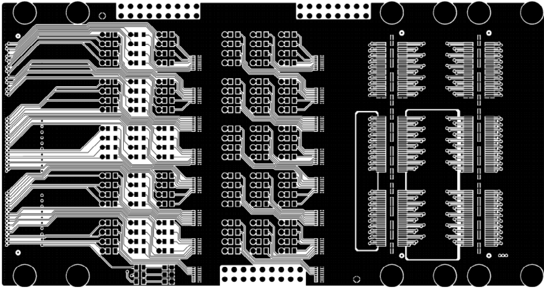
TOP LAYER
