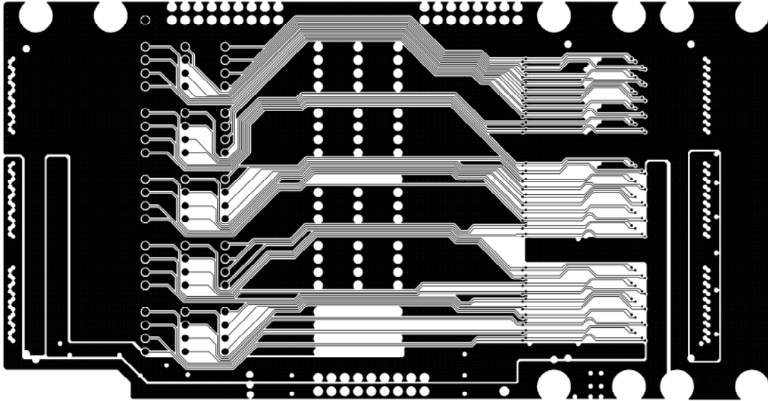
MID LAYER1
