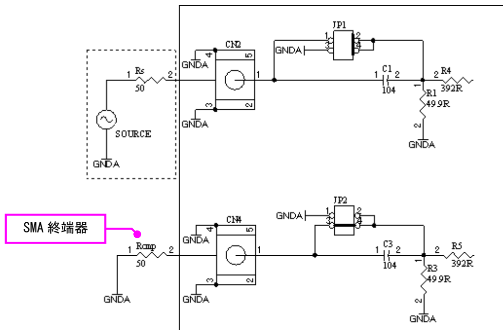
シングルエンド入力時の推奨設定
