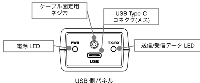
USB 側パネル
