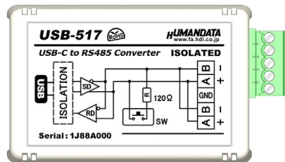
上面 (銘板)
