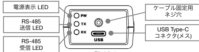
USB 側パネル
