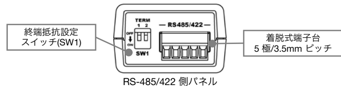
RS-485/422 側パネル
