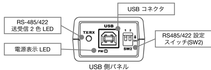
USB 側パネル
