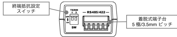
RS-485/422 側パネル
