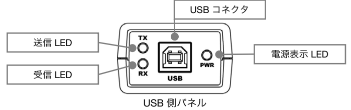
USB 側パネル
