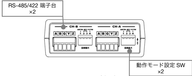
RS-485/422 側パネル
