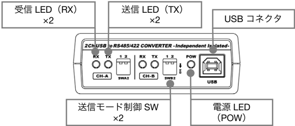
USB 側パネル
