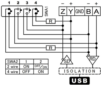
チャンネル A 接続図
