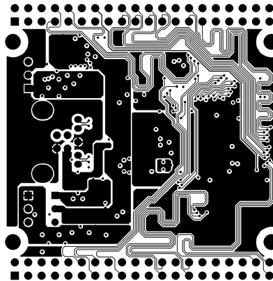
BOTTOM LAYER
