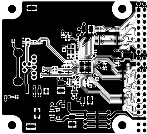
TOP LAYER
