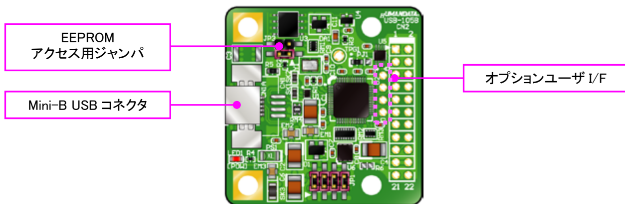
部品面 (USB-105-M)
