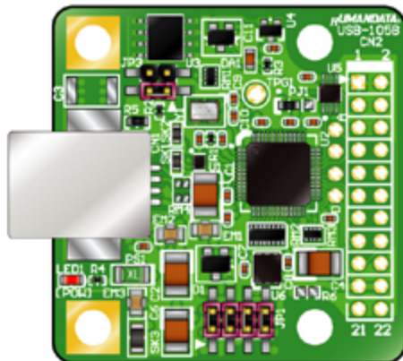
USB-105-S
