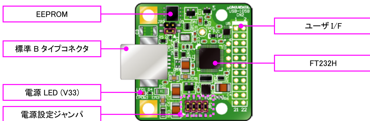
部品面 (USB-105-S)
