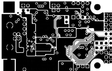
BOTTOM LAYER
