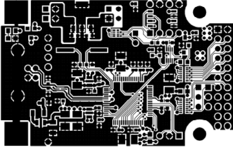
TOP LAYER
