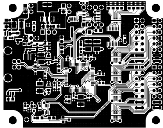
TOP LAYER
