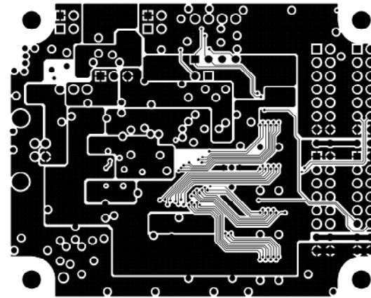
BOTTOM LAYER
