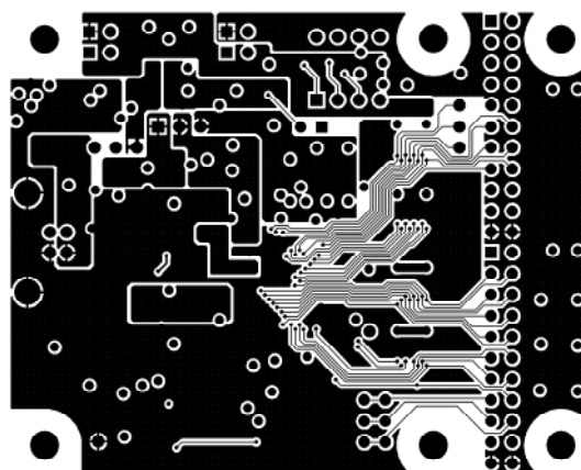
BOTTOM LAYER
