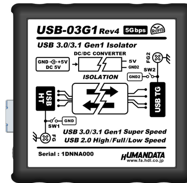
上面 (銘板)
