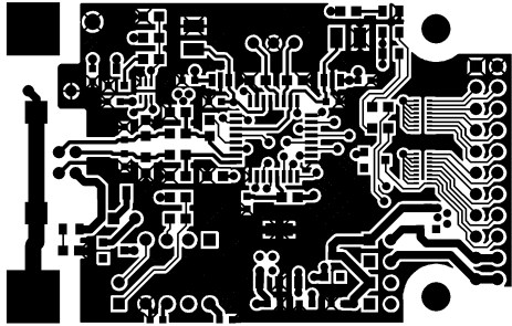
TOP LAYER
