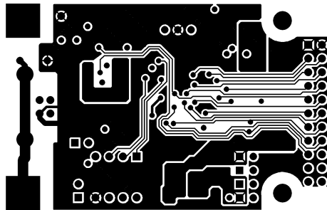
BOTTOM LAYER
