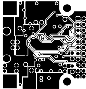
BOTTOM LAYER
