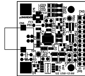
部品面
